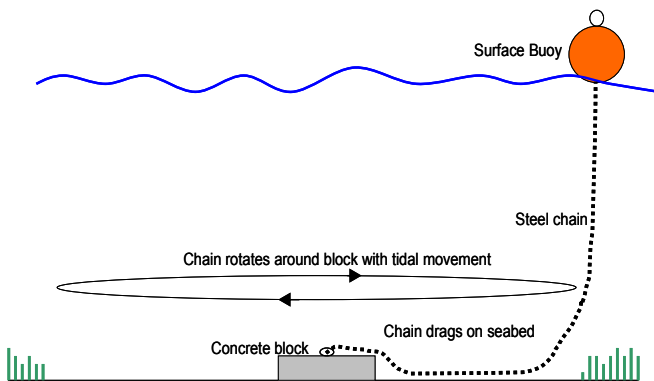
Ffigwr 2: Dyluniad system angori arferol a sut y mae'n cael ardrawiad ar wely'r môr
